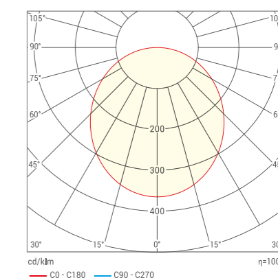
Косинусная КСС
