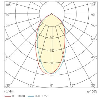
Асимметричная КСС (А50)
