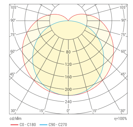
Косинусная КСС
