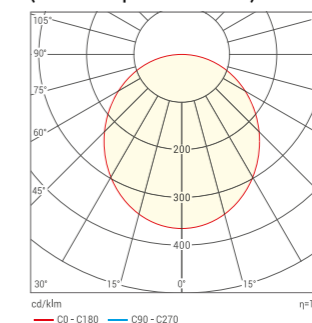
Косинусная КСС (матовый рассеиватель)
