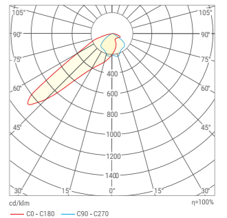
Косинусная КСС (Д90)
