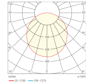
Косинусная КСС (Д120)
