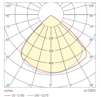
Концентрированная КСС (К30)
