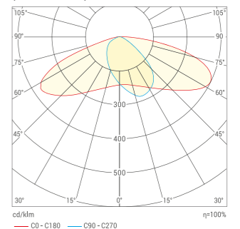
Широкая Боковая КСС (ШБ156x68)
