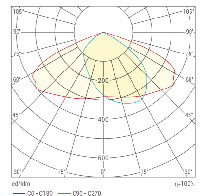
Широкая Боковая КСС (ШБ130x75)
